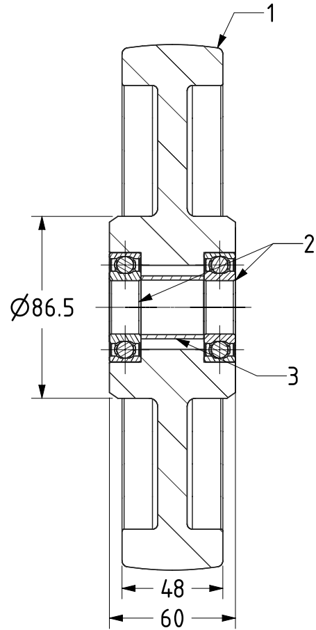
SECTION A-A
