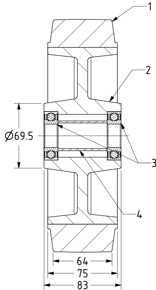
SECTION A-A
