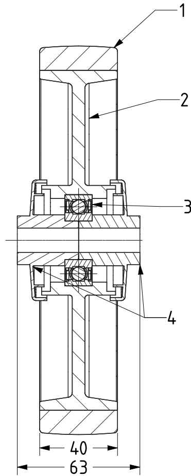
SECTION A-A
