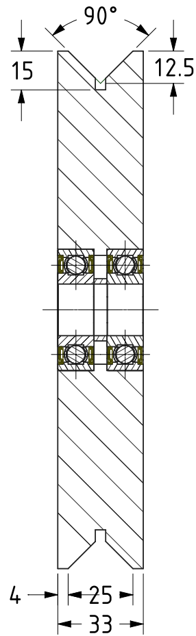
SECTION A-A
