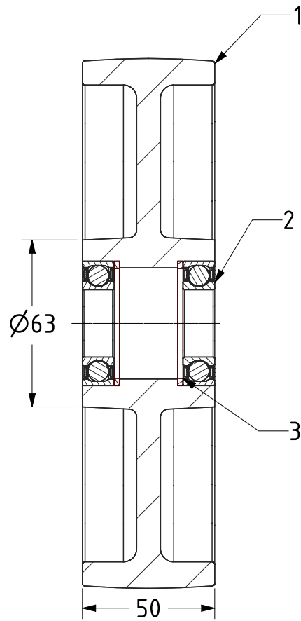
SECTION A-A
