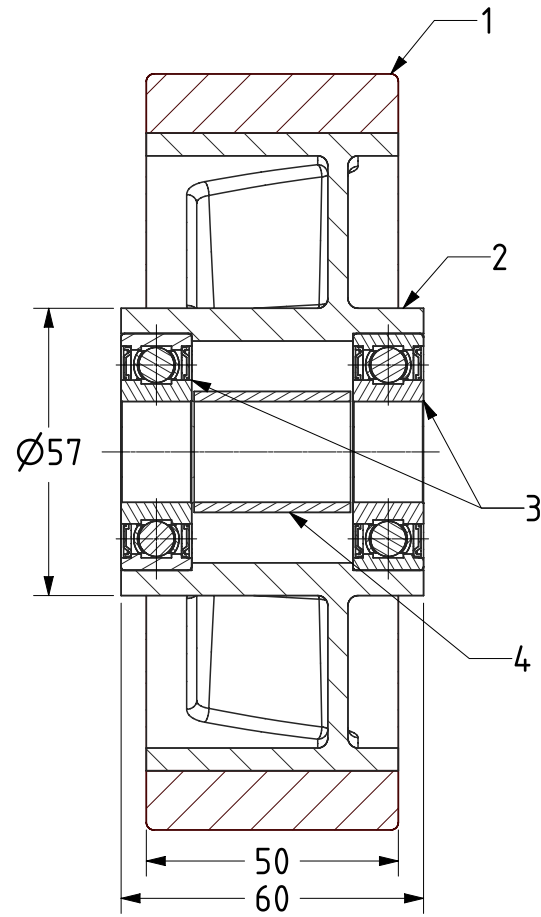
SECTION A-A
