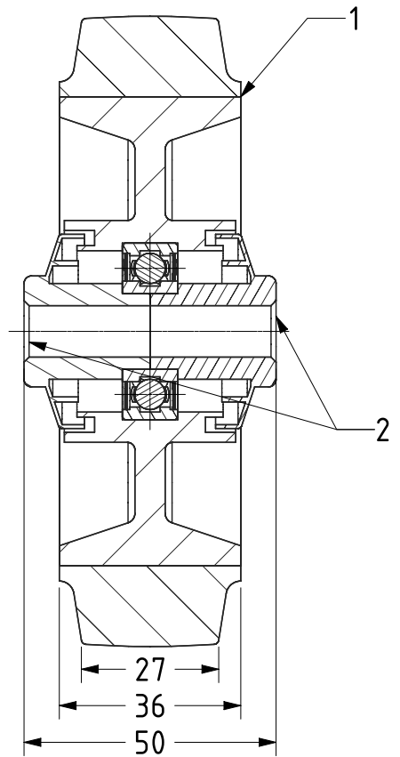
SECTION A-A
