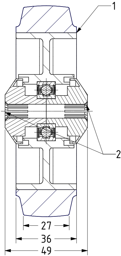
SECTION A-A
