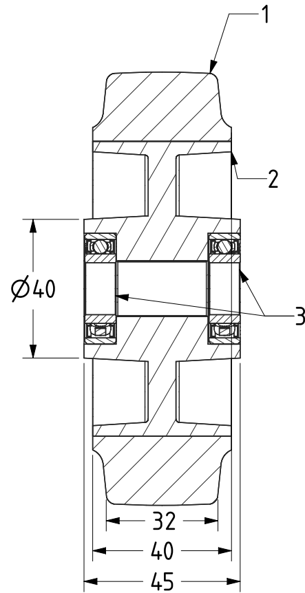
SECTION A-A
