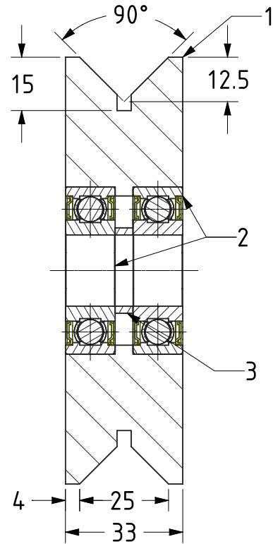
SECTION A-A
