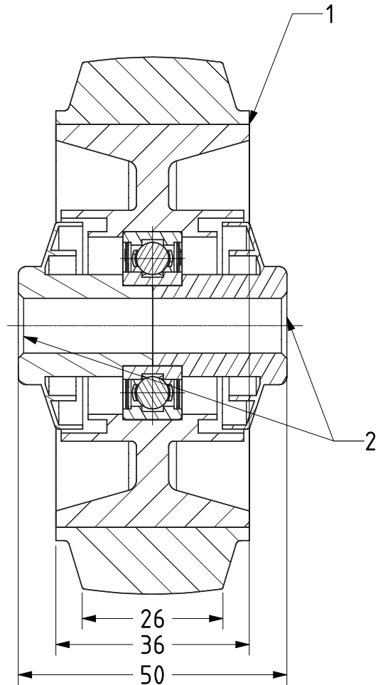
SECTION A-A
