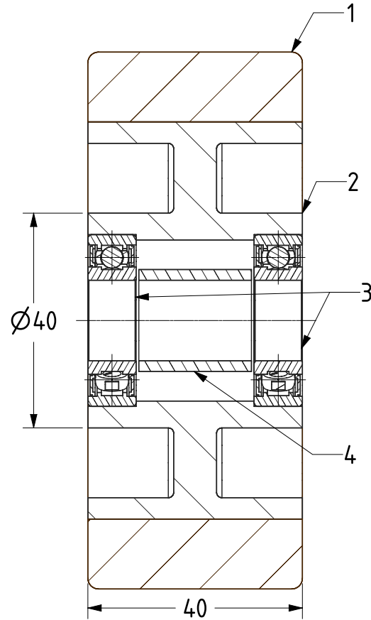
SECTION A-A
