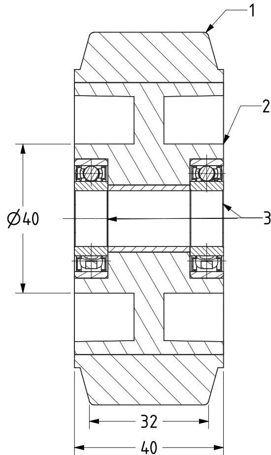
SECTION A-A
