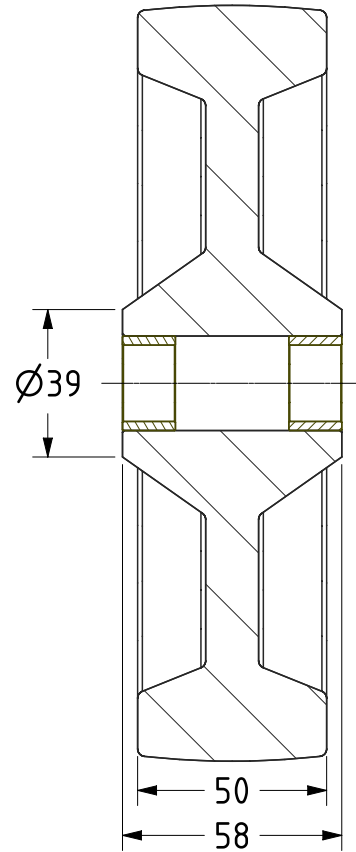
SECTION A-A
