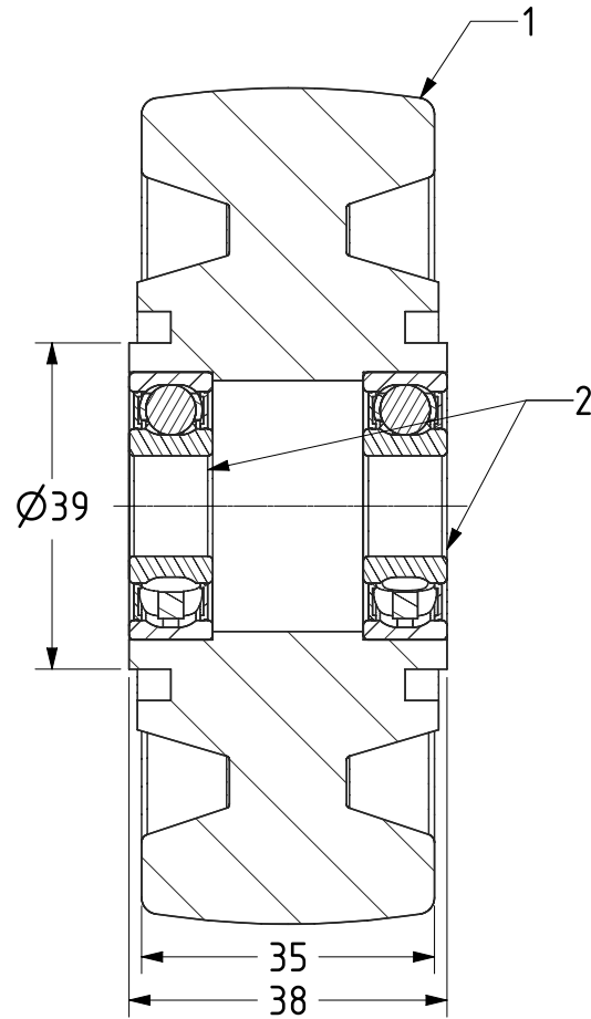
SECTION A-A
