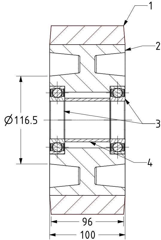
SECTION A-A
