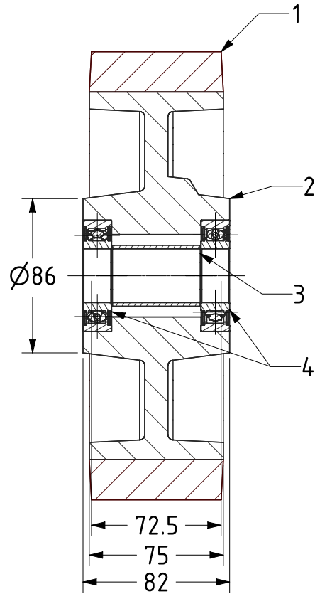
SECTION A-A
