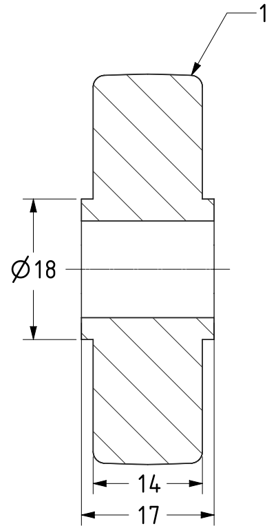
SECTION A-A
