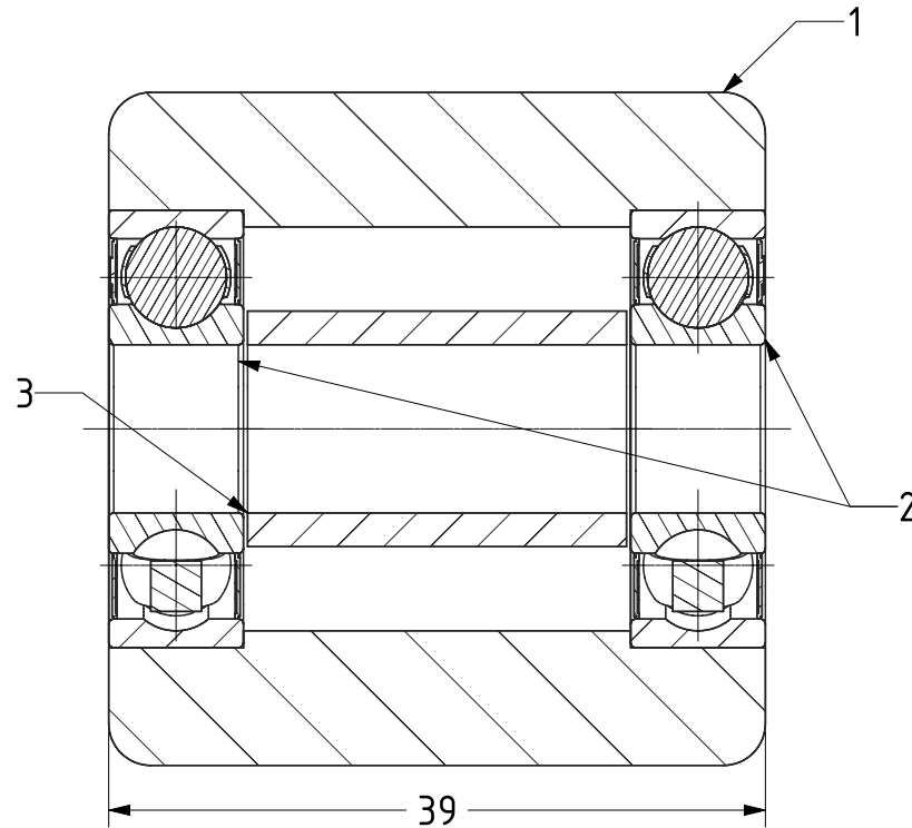
SECTION A-A
