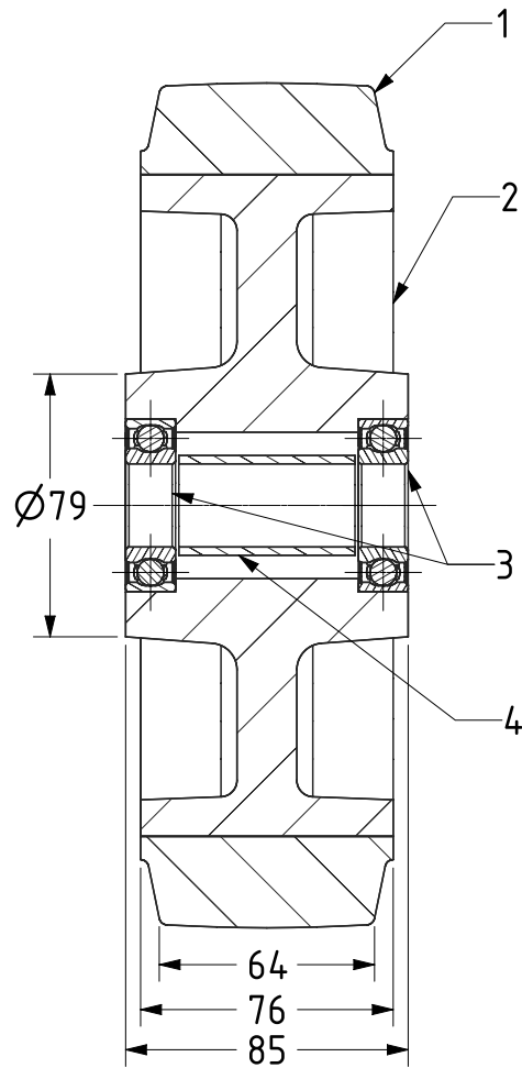
SECTION A-A
