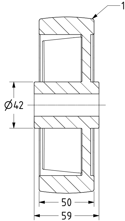
SECTION A-A
