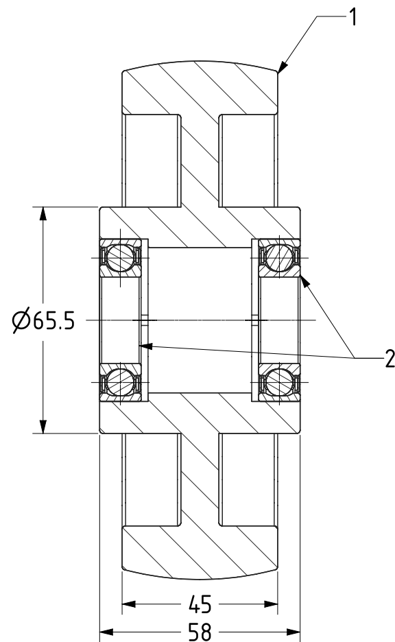
SECTION A-A
