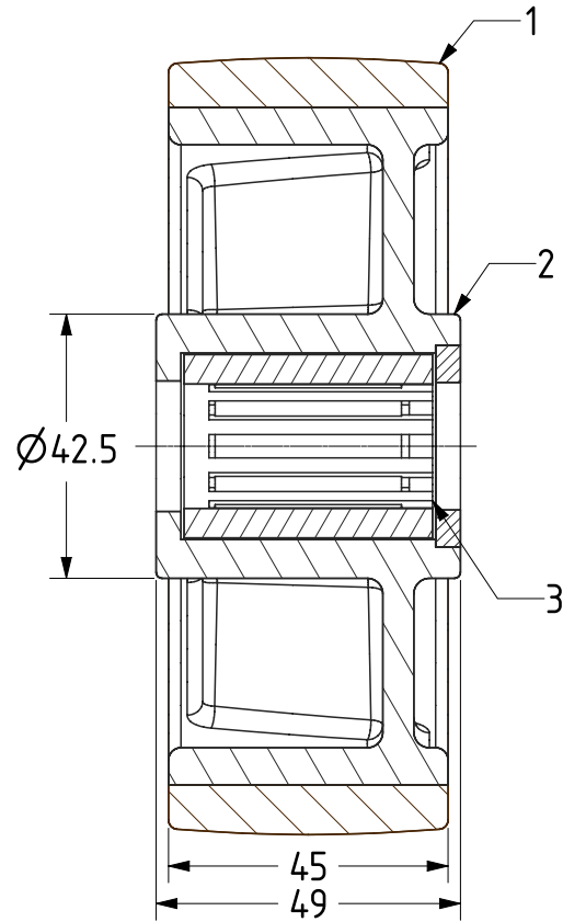
SECTION A-A
