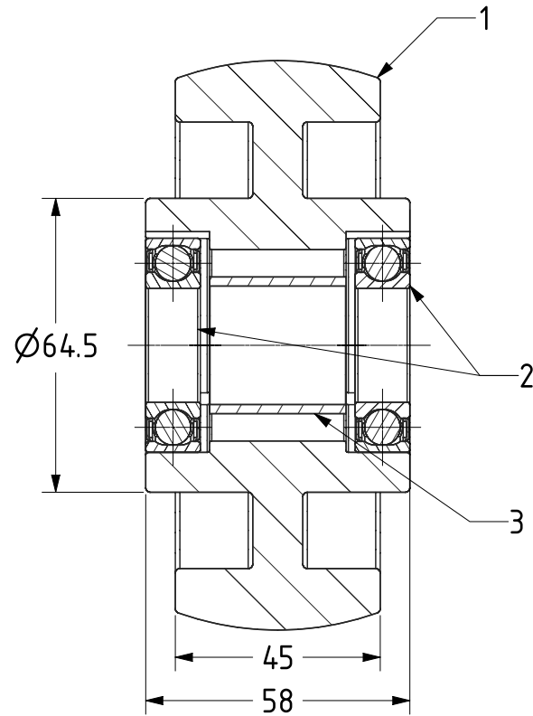
SECTION A-A
