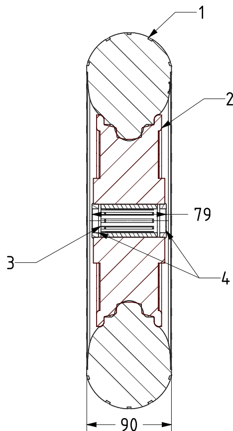
SECTION A-A
