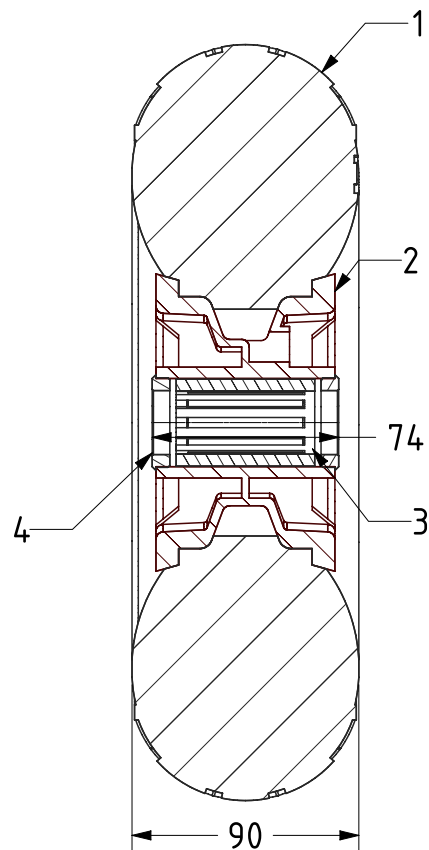
SECTION A-A
