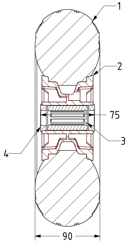
SECTION A-A
