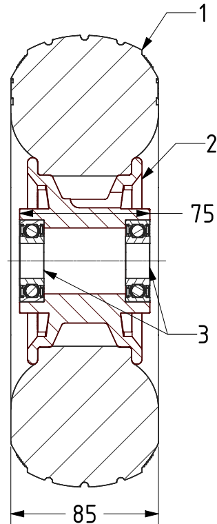
SECTION A-A
