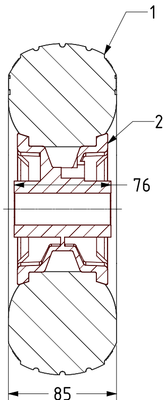
SECTION A-A
