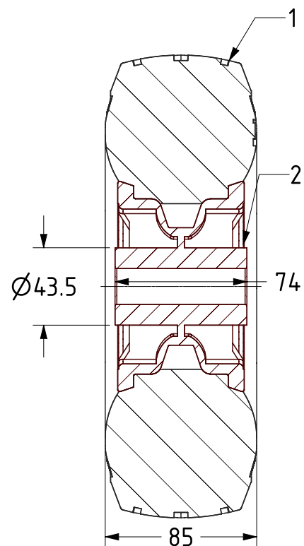
SECTION A-A
