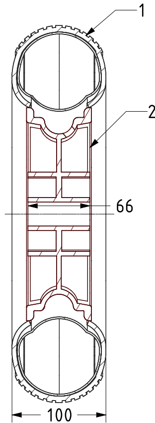
SECTION A-A
