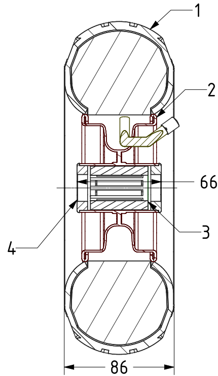
SECTION A-A
