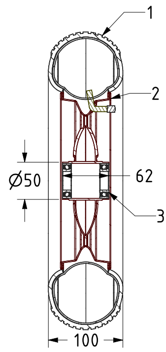
SECTION A-A
