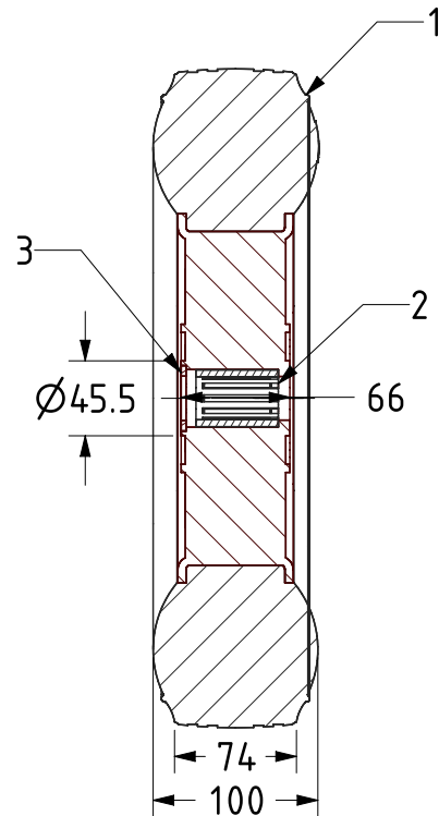
SECTION A-A
