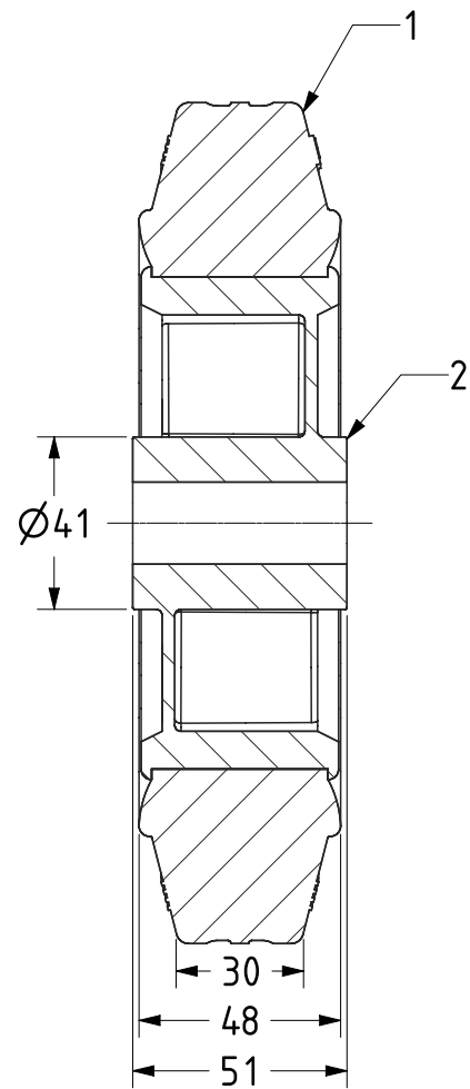
SECTION A-A
