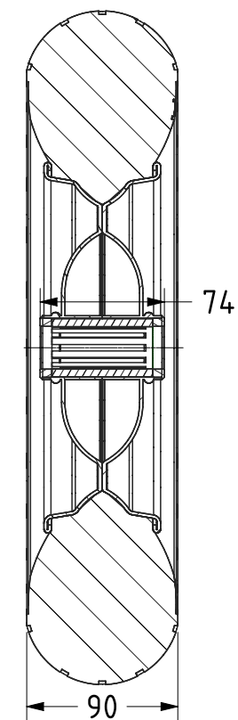
SECTION A-A
