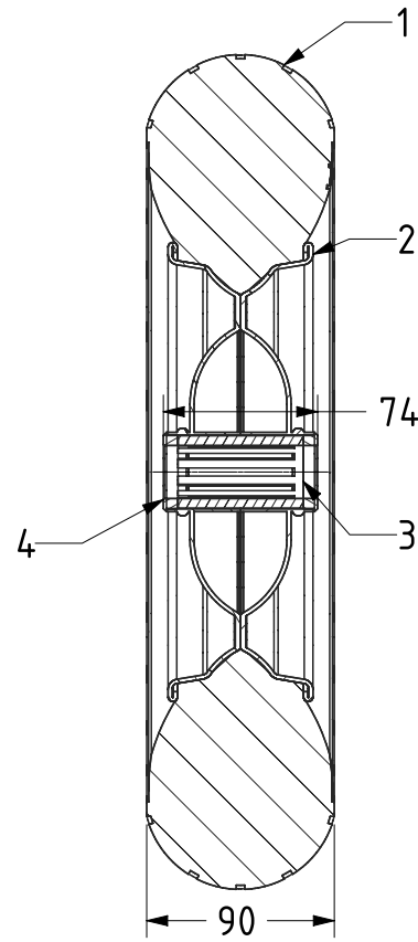
SECTION A-A
