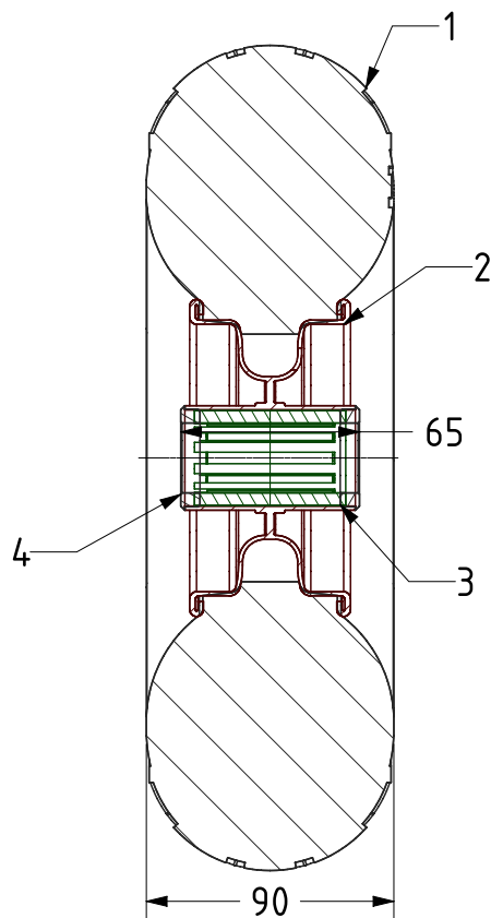
SECTION A-A
