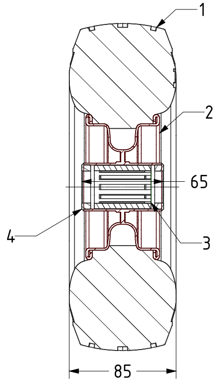
SECTION A-A
