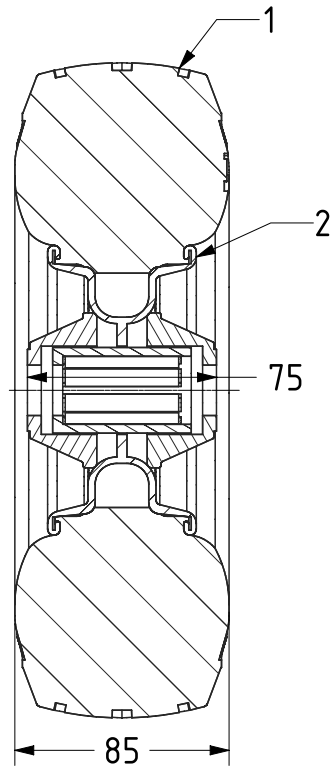
SECTION A-A
