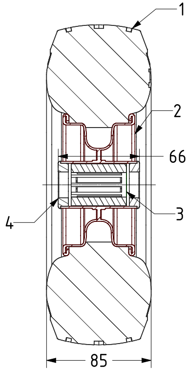
SECTION A-A
