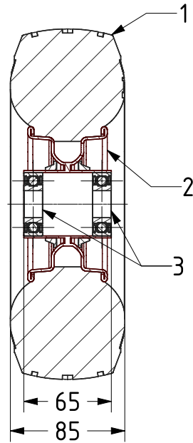
SECTION A-A
