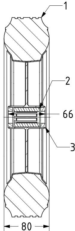
SECTION A-A
