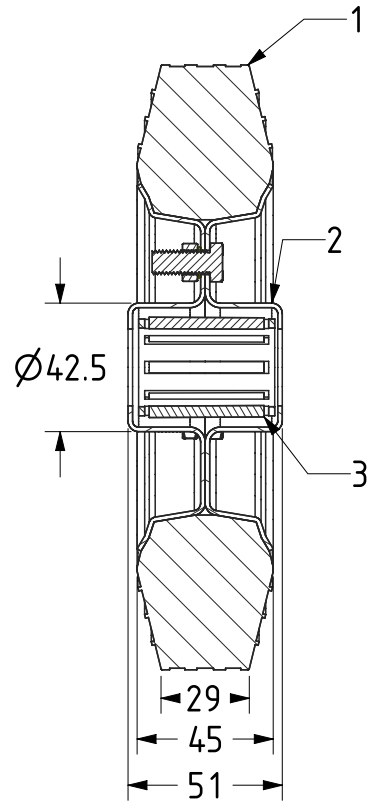
SECTION A-A
