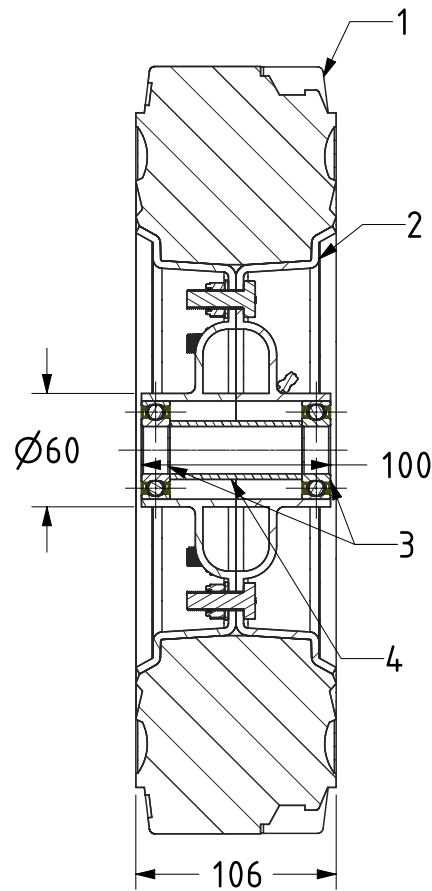
SECTION A-A
