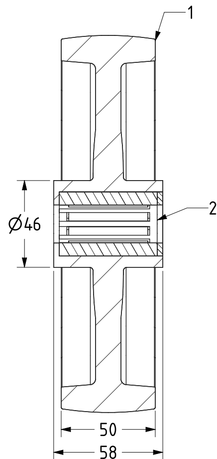
SECTION A-A
