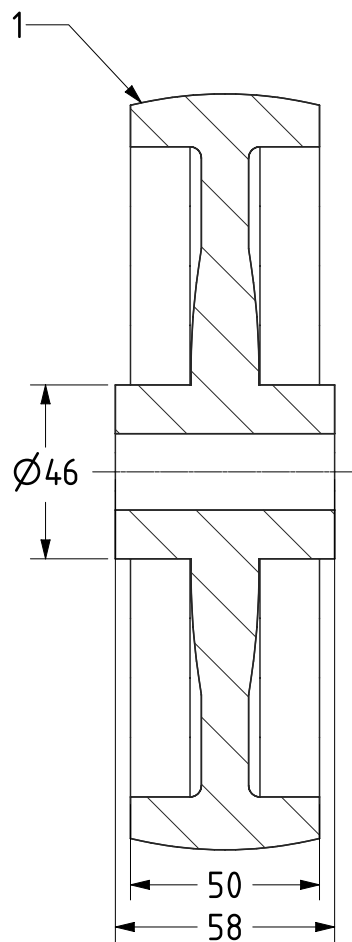
SECTION A-A
