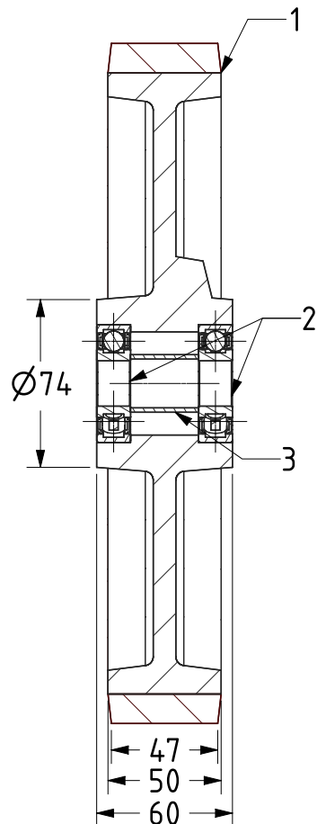
SECTION A-A
