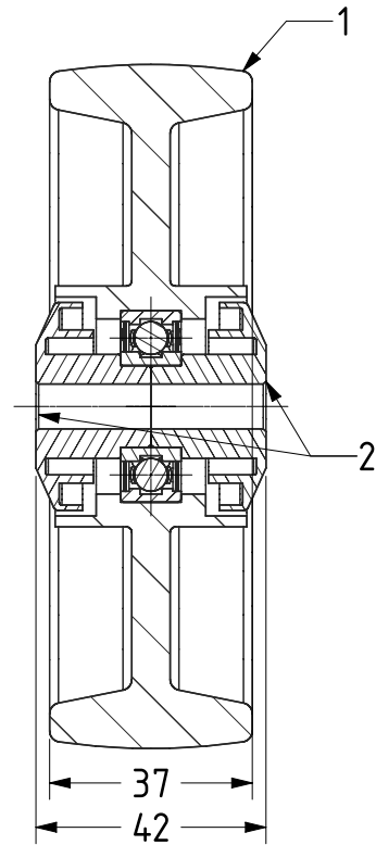
SECTION A-A
