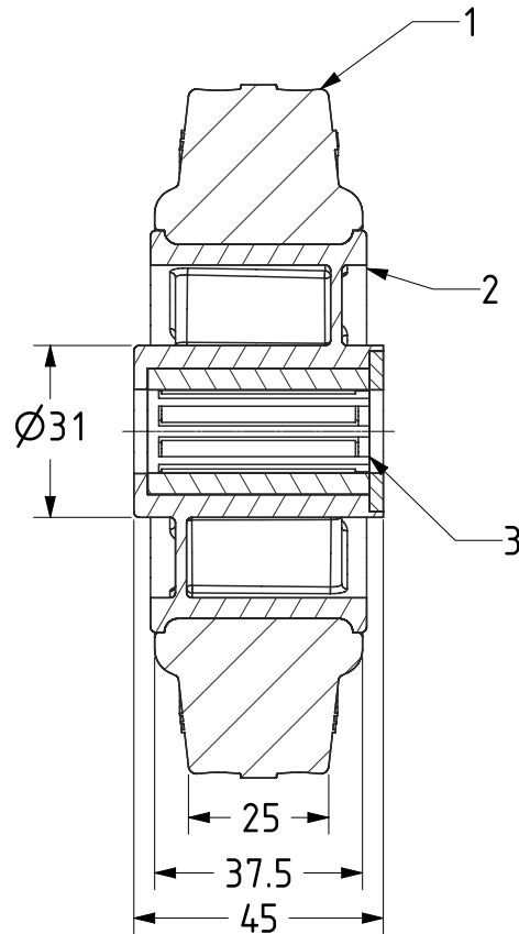
SECTION A-A
